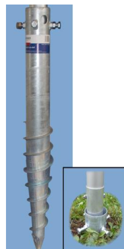
Aluminium-Bodenhülse im Schraubfundament
